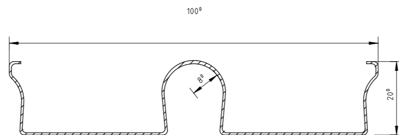
Schnitt Front
